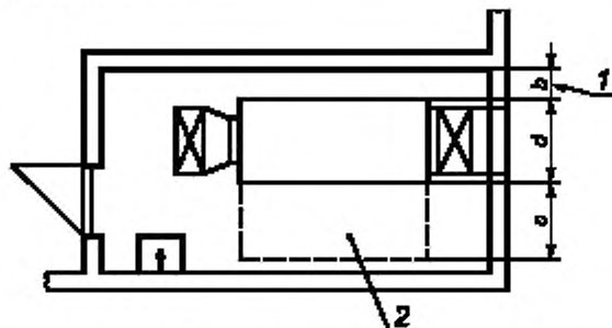
Рисунок А.5 — Расположение кондиционера (в плане)
