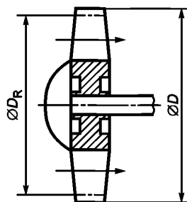
Рисунок 2 — Рабочее колесо осевого вентилятора
