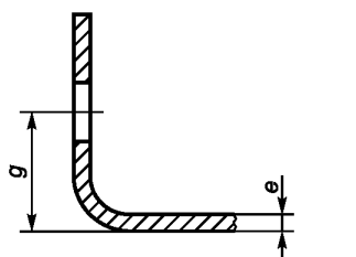
Катаный фланец
