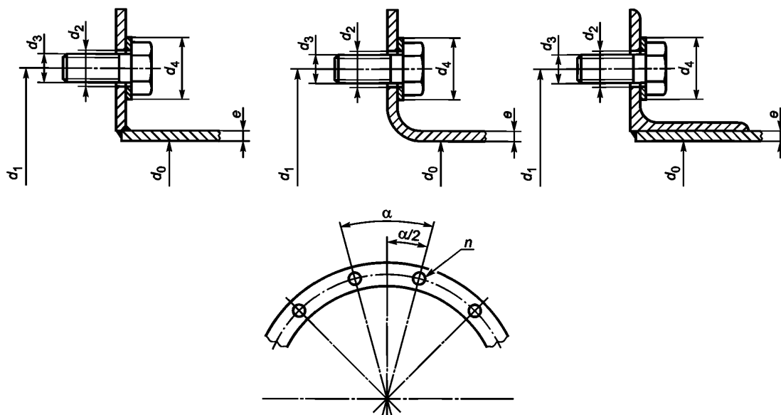
Рисунок 4 — Размеры круглых фланцев
