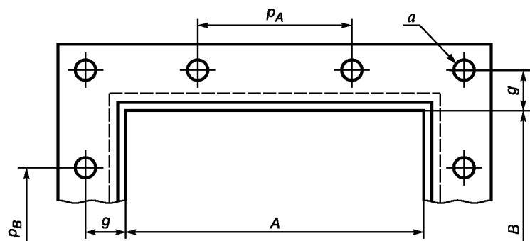
Приваренный внахлест фланец
