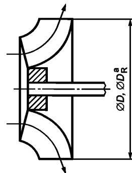
Рисунок 3 — Рабочее колесо диагонального вентилятора
