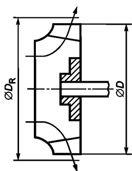
Рисунок 1 — Рабочее колесо радиального вентилятора
