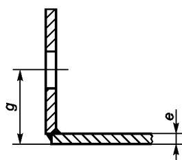
Сварной фланец
